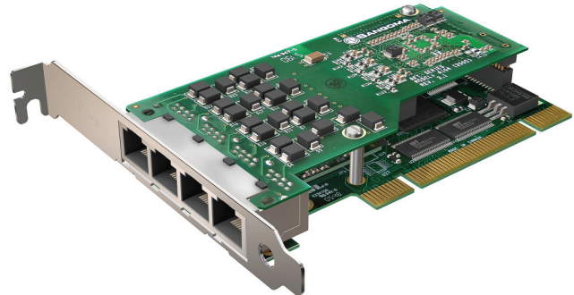
Placa A104 de 04 portas E1/T1/J1 de interface com barramento PCI.
